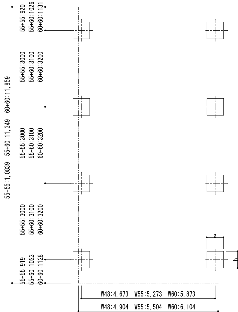
■ 基礎配置図
