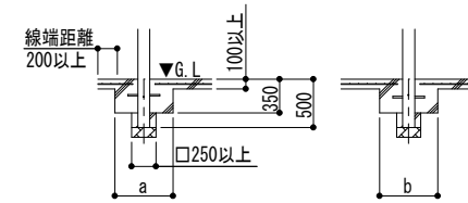
■ 基礎断面図
